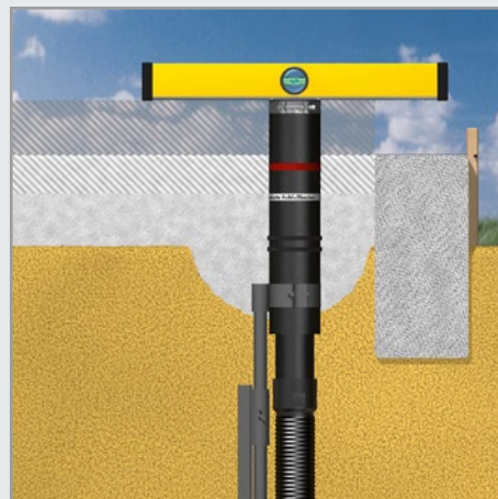
Abb. 16: Ausrichtung Quadro-Secura® E-BP-R
