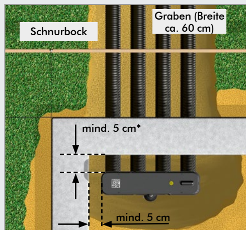
Abb. 11: Platzierung Quadro-Secura® Basic-FUBO-E-R4+
