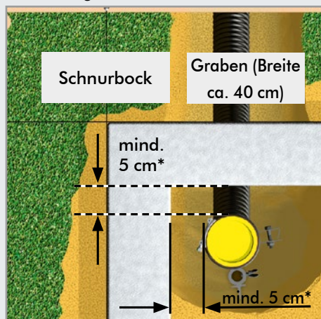
Abb. 15: Platzierung Quadro-Secura® E-BP-R
