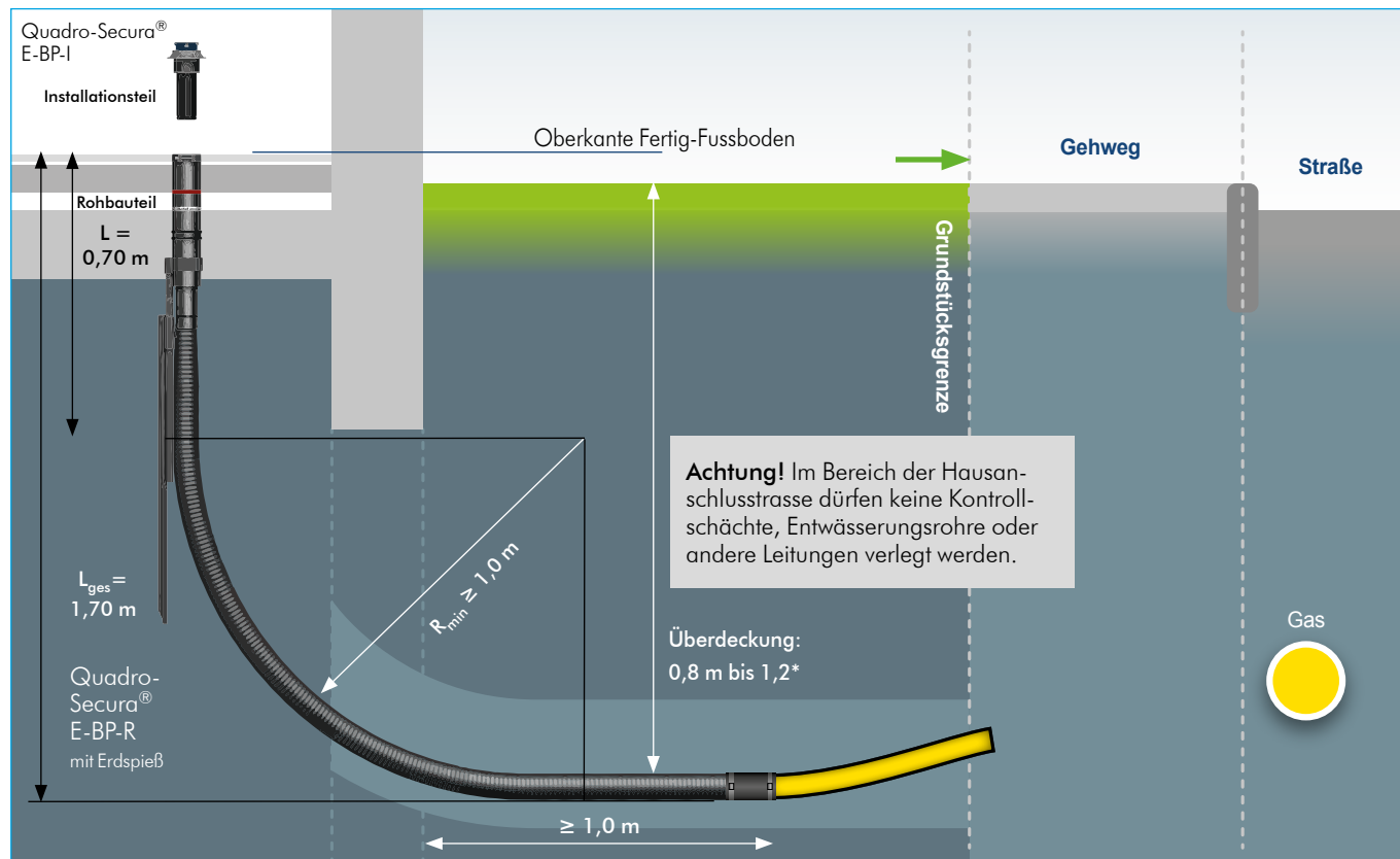
Abb. 14: Einbau Quadro-Secura® E-BP
