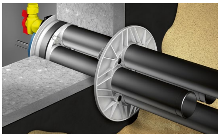
Quadro-Secura® Nova 1
